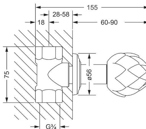
mit Einbaukörper 3/4"
