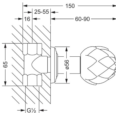
mit Einbaukörper 1/2"
