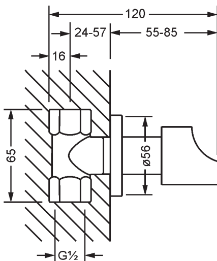
mit Einbaukörper ½"
