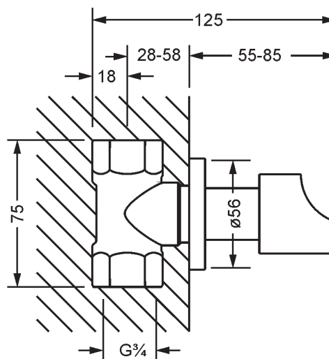
mit Einbaukörper ¾"
